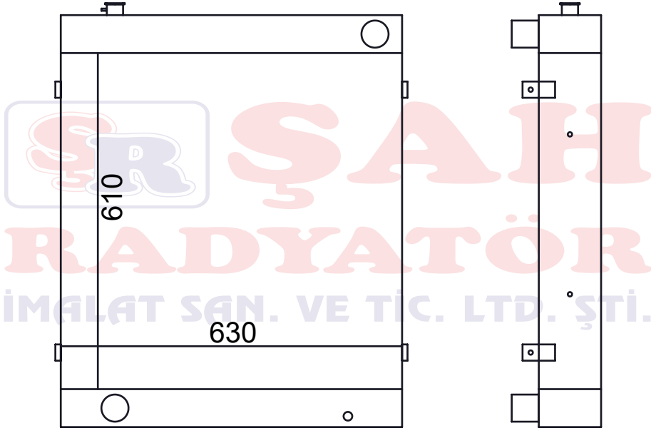
JCB 415
